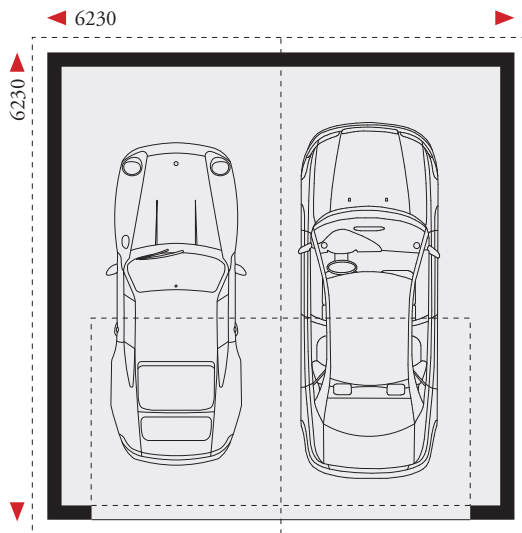
GARAŻ 34,22 m 2 garaż dwustanowiskowy, dach dwuspadowy, brama od szczytu
