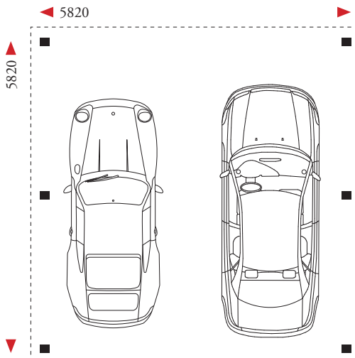
WIATA GARAŻOWA 33,87 m 2 wiata garażowa dwustanowiskowa, dach jednospadowy
