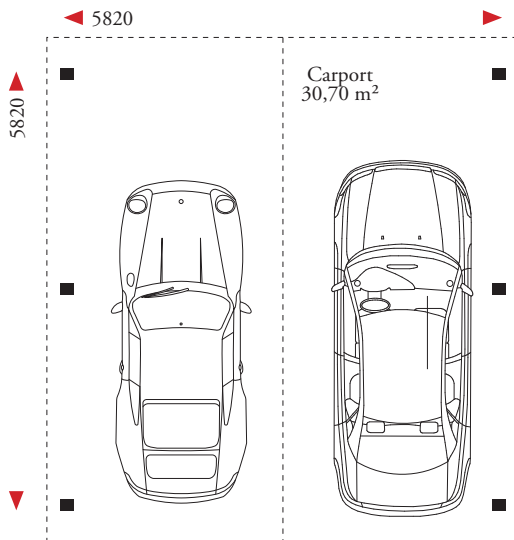
CARPORT 30,70 m 2 carport dwustanowiskowy, dach dwuspadowy
